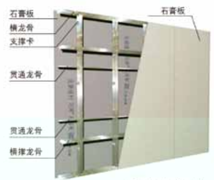
有贯通龙骨隔墙示意图
